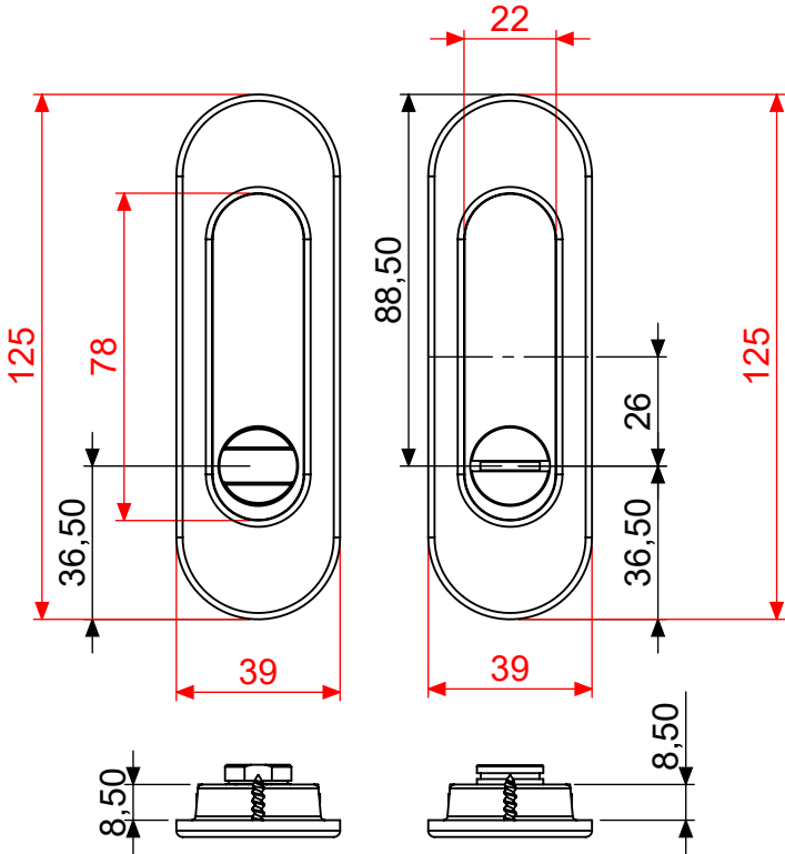
placca incasso noxia scala 1:2
