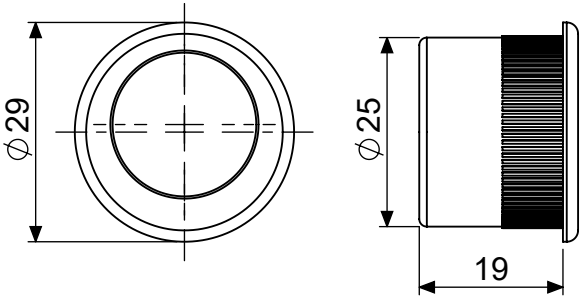
frontale incasso scala 1:1
